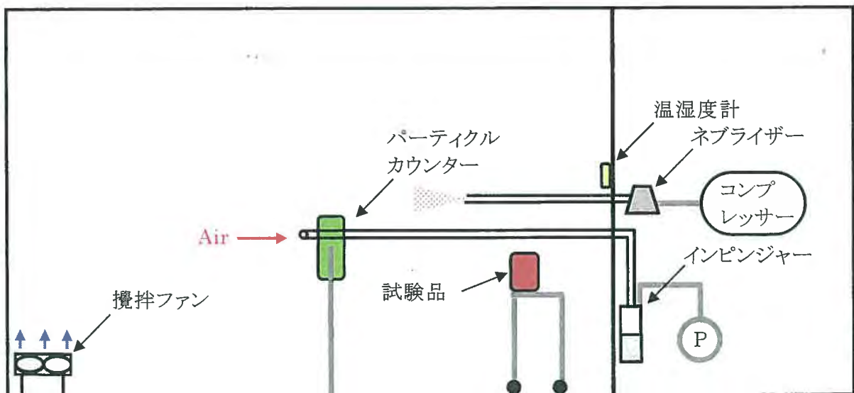
別紙図 c. 25 m 3 試験チャンバーの外観 (側面図)
